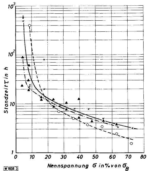
Abb. 3. Abhängigkeit der Standzeit \tau der molybdänhaltigen Stähle D bis F in siedender, 42%iger Magnesiumchlorid-Lösung von der Spannung \sigma x — x Stahl D o — o Stahl E Δ — Δ Stahl F
