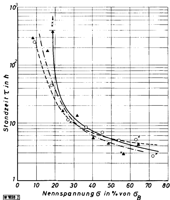
Abb. 2. Abhängigkeit der Standzeit \tau der molybdänfreien Stähle A bis C in siedender, 42%iger Magnesiumchlorid-Lösung von der Spannung \sigma x — x Stahl A o — o Stahl B Δ — Δ Stahl C
